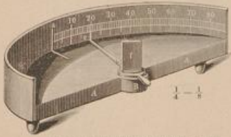
Fig. 2. Apparat zum Nachweis der Reflexionsgesetz.
