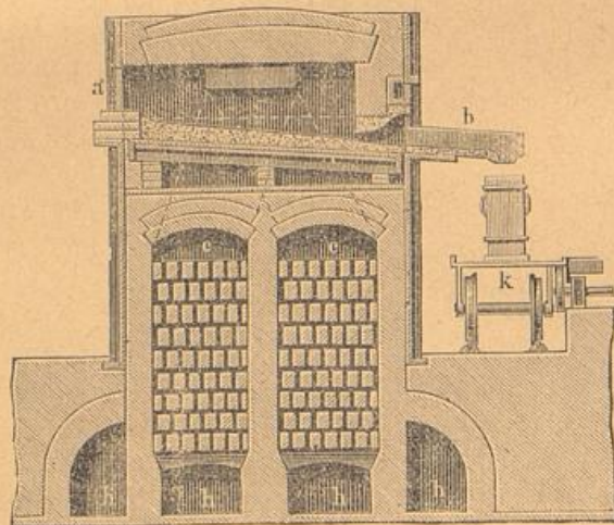
Fig. 2. Querschnitt.
