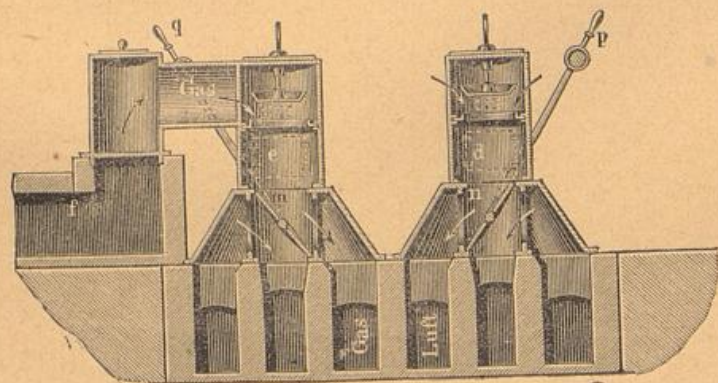
Fig. 3. Reversir-Apparat. Ein Siemens-Martinofen (f. Stahl) mit Regenerativgasfeuerung.
