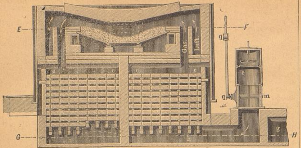
Fig. 1. Längsschnitt.
